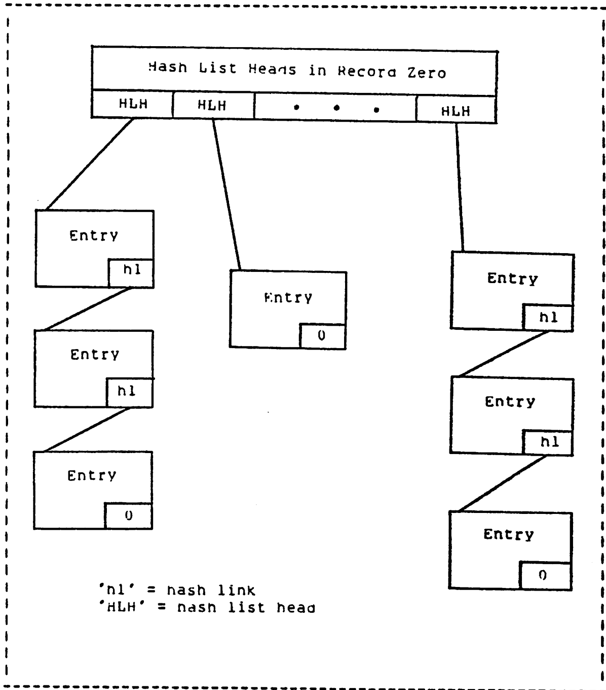
Illustration 3.4.1.4 -- Hash Lists
